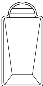
MALAGA L 9,60 m x l 4,20 m Petit bain 1,10 m Grand bain 1,90 m
